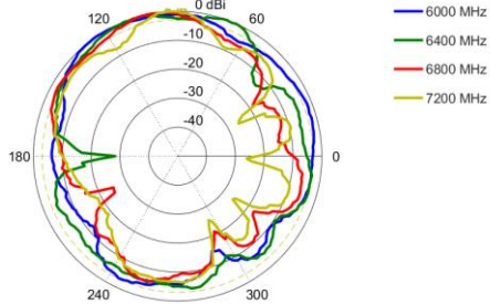
Elevation 2: 6000 – 7200 MHz
