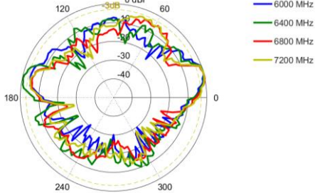
Elevation 2: 6000 – 7200 MHz
