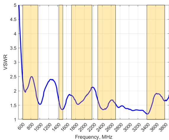
VSWR
