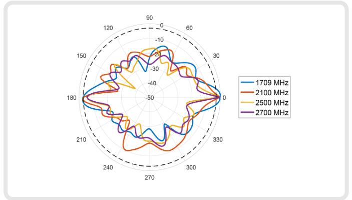
E-Plane: 1700 - 2700 MHz
